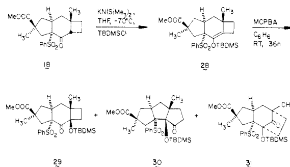
Scheme VI
